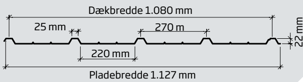
DS Pandeplade 22-270 med spor
